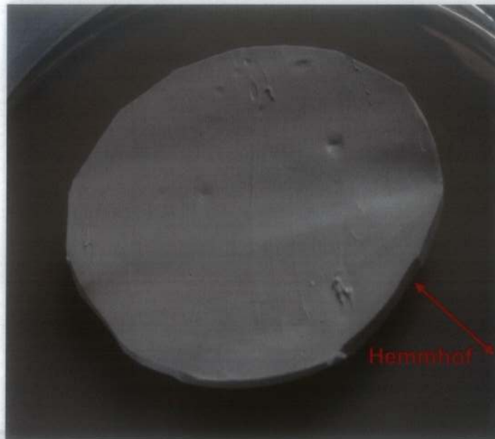
Foto 1: Untersuchungsmaterial Soudaseal Cleanroom nach einer Inkubationszeit von 28 Tagen ohne sichtbaren Pilzbewuchs mit Hemmhof um den Prüfkörper herum
